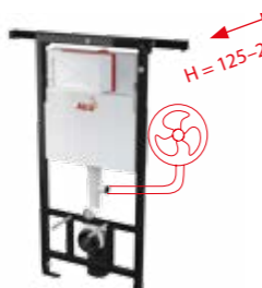
AM102/1120V Jádromodul Falsík alatti szerelési rendszer szellőző előkészítéssel száraz szereléshez (főképp panellakások fürdőszobáinak átépítéséhez)
