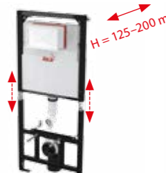
AM101/1120D Sádromodul Szétvehető falsík alatti szerelési rendszer száraz szereléshez (gipszkarton)
